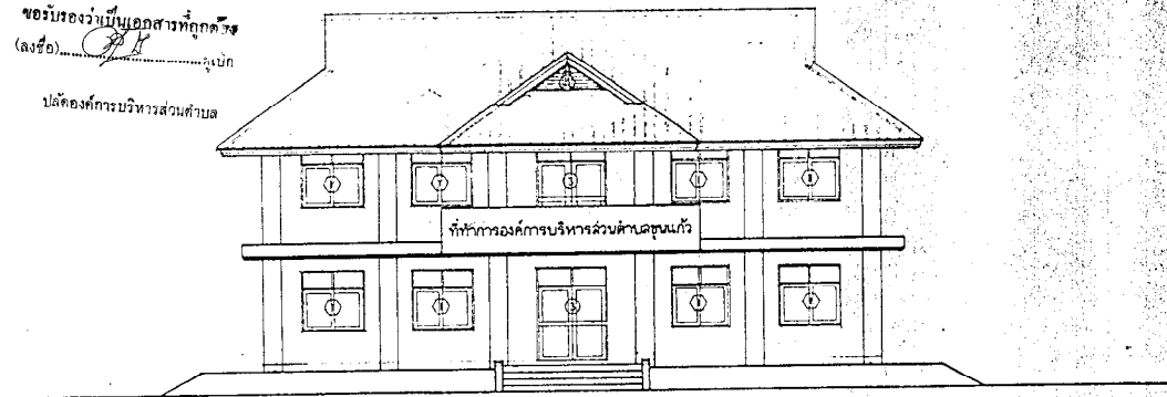
รูปด้าน 1. 1:100
